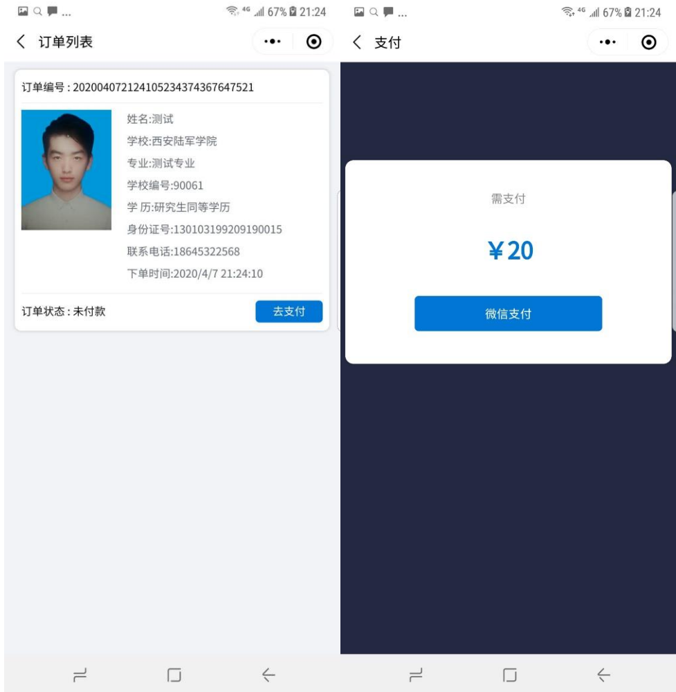
订单界面
