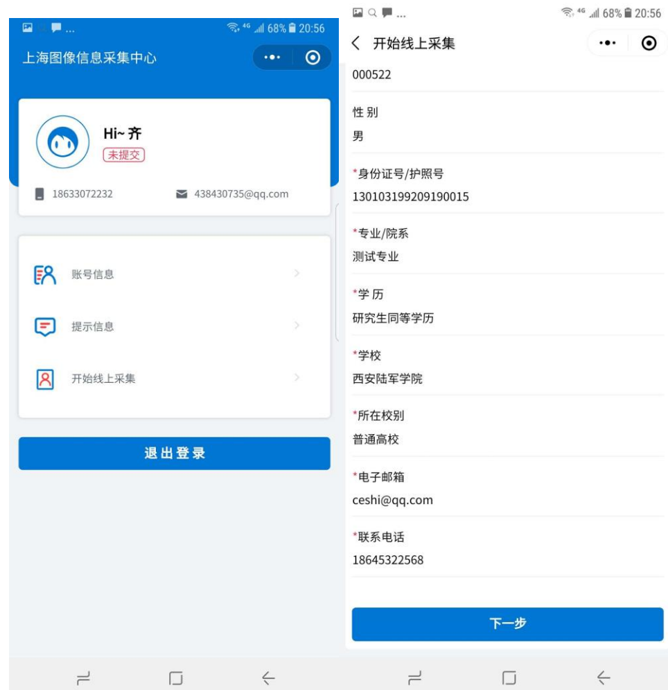
系统主界面
